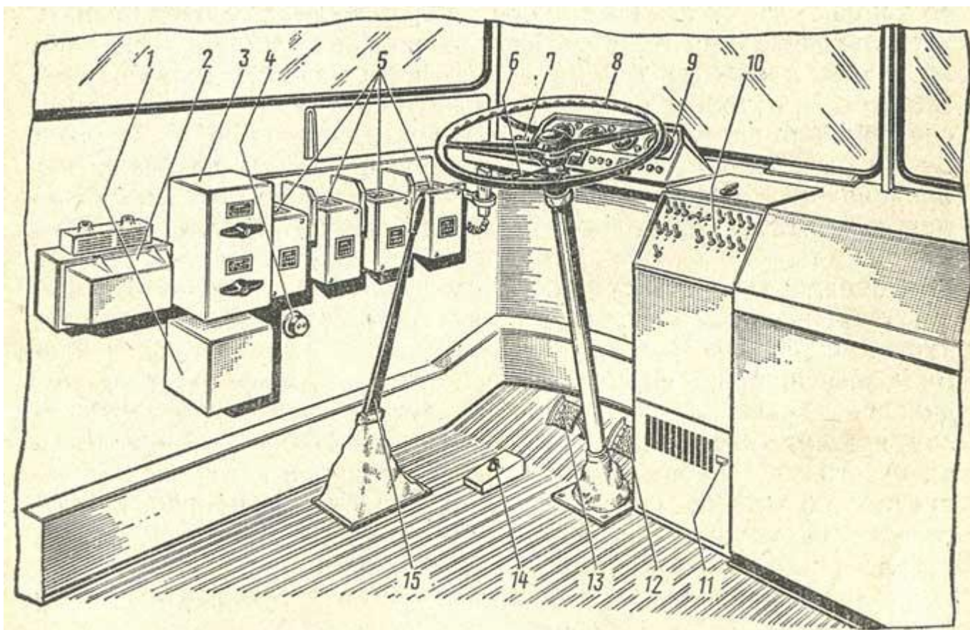
Рис. 159. Кабина водителя:
