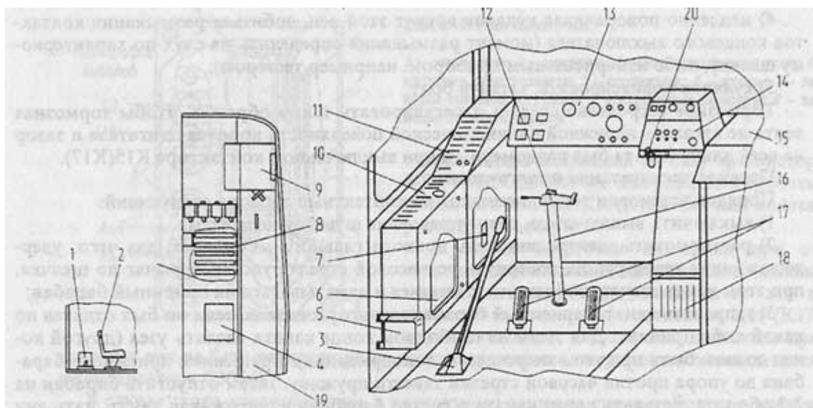
Рис. 6.11. Расположение аппаратов в кабине водителя:
